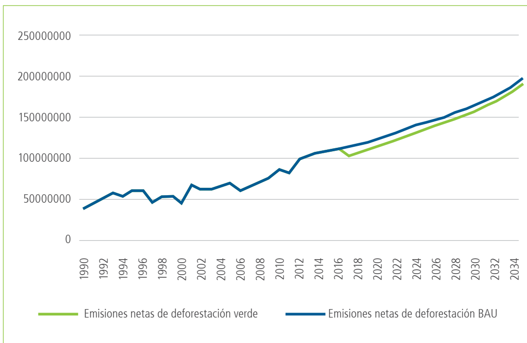
Gráfico 4: Emisiones netas provenientes por deforestación (CO2eq) por escenario 1990-2035
